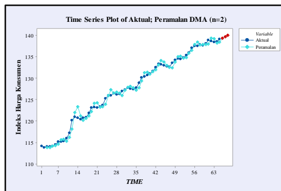
Gambar 2: Grafik perbandingan hasil peramalan dengan data aktual
