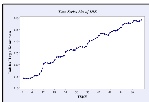
Gambar 1: Grafik runtun waktu IHK Kota Samarinda
